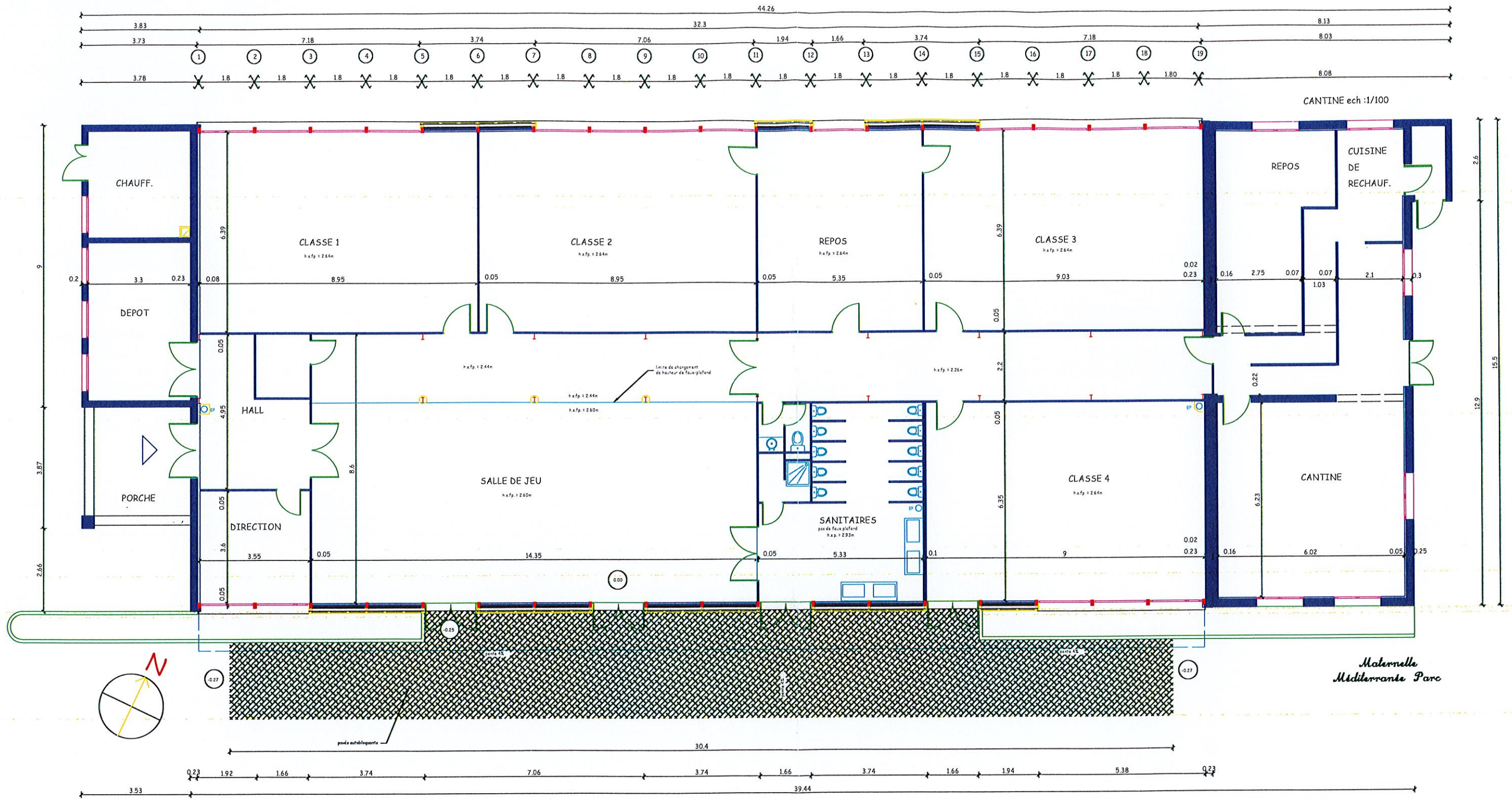
Plan intérieur - Ecole Maternelle Parc Méditerranée
